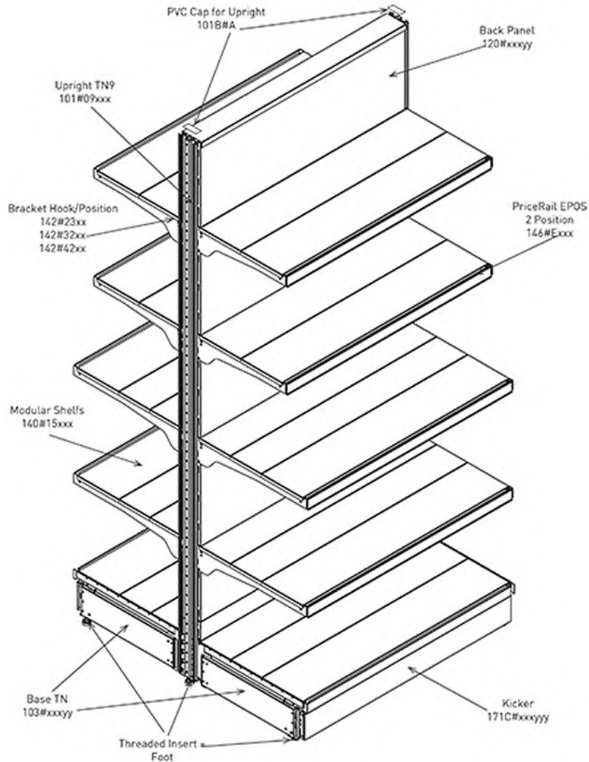
R-Series Gondola
